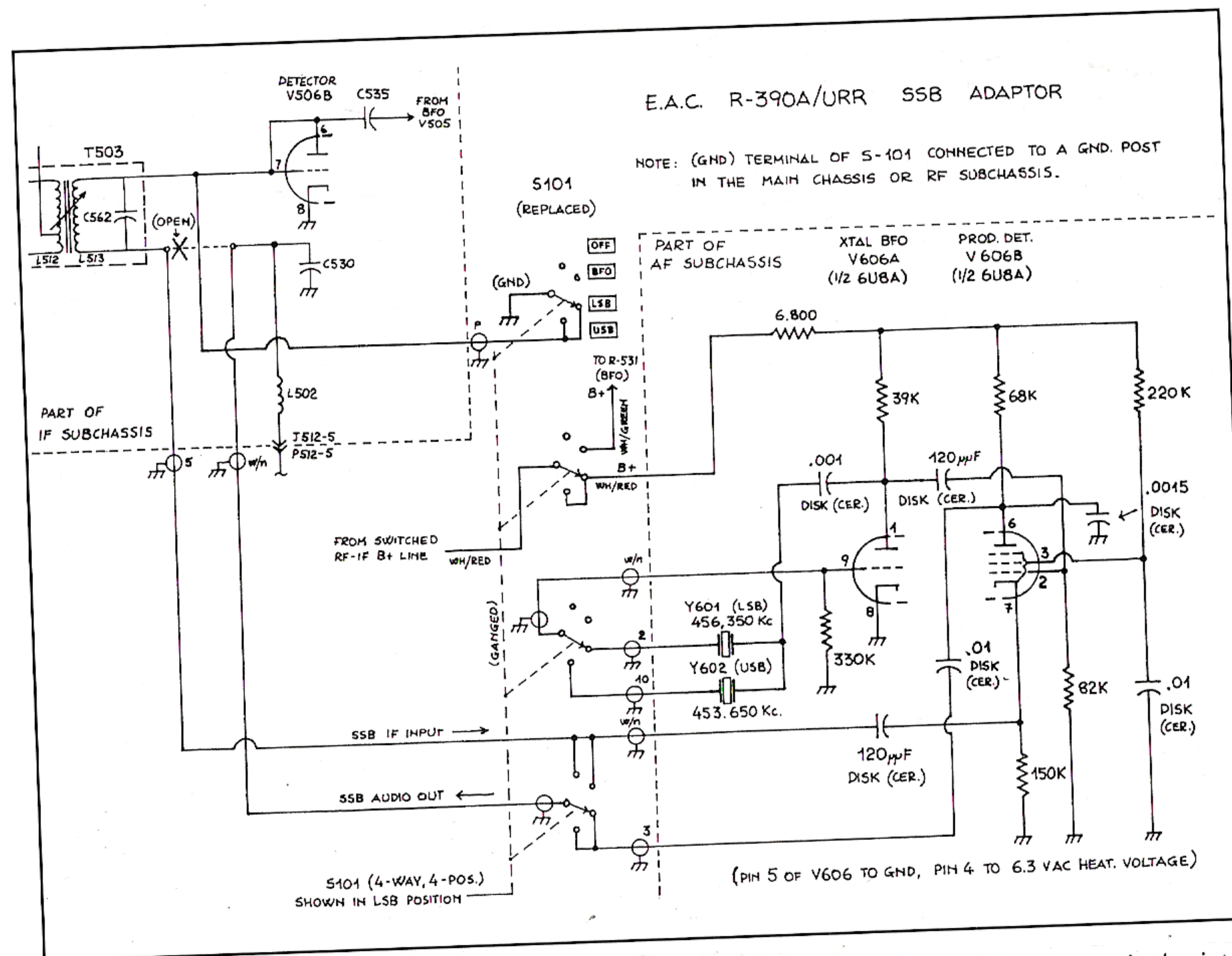
Fig. 23 - Schema elettrico dei circuiti relativi al rivelatore a prodotto installato dall'Electronic Assistance Co.
